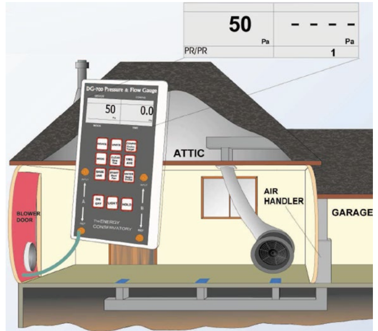
Figura 1: Prueba 2 de Fuga de Ductos al Exterior
